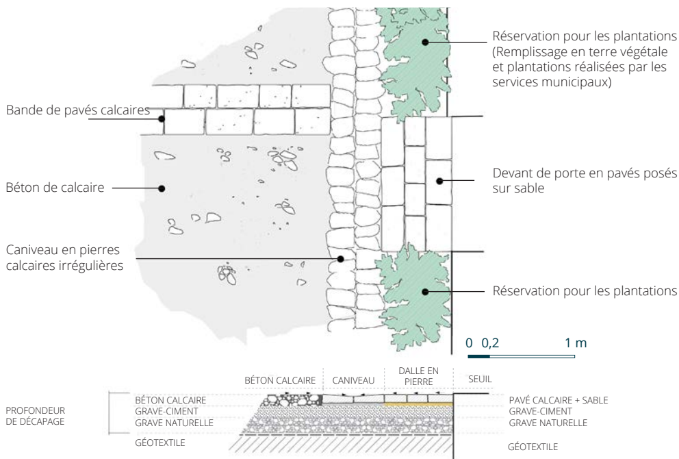
Détail du caniveau latéral
