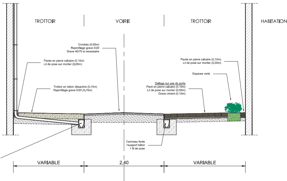
Coupe type de voirie
