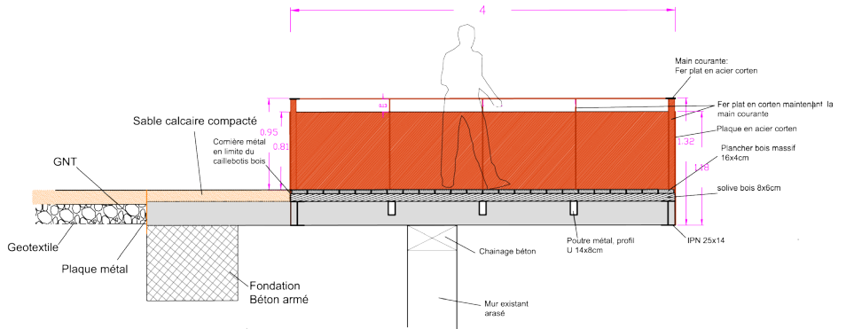
Coupe technique du belvédère
